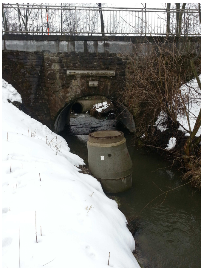
Propustek pod ulicí U Potoka s kanalizační šachtou – místo omezující odtokové poměry (směr po toku)
